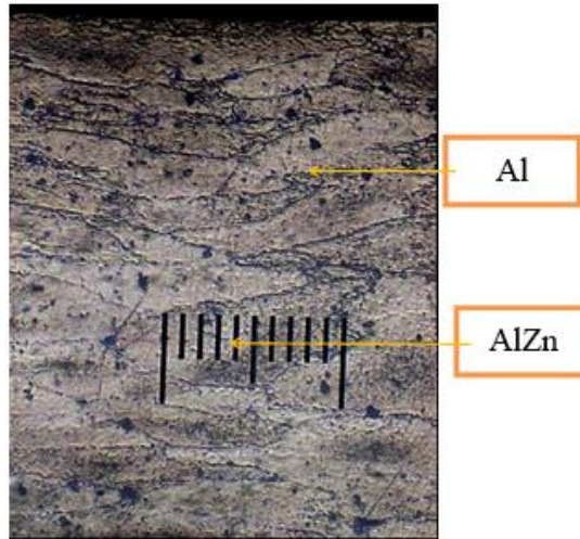
Gambar 3. Struktur mikro Al-Zn dengan proses cold rolling perbesaran 100x.
